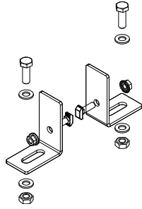
CCR-L Askı Takımı ("T" cıvatalı)
