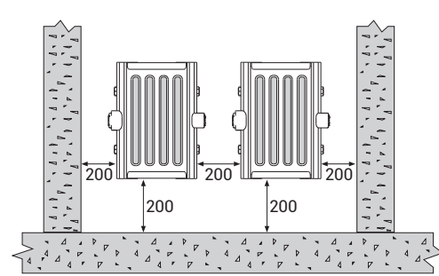
Şekil 8 - Galeri Dikey Pozisyon
