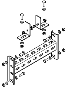
CCR-UT Askı Takımı ("T" cıvatalı)
