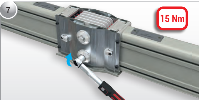
Somun kilitleme kapakları yeniden takılır ve 15Nm ile torklanır.
