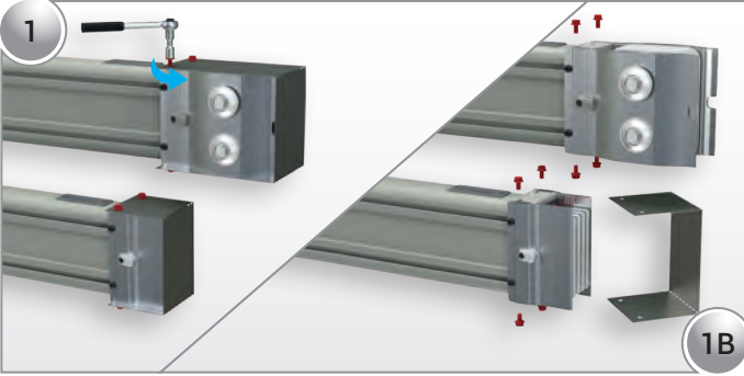
Cıvatalar sökülerek busbar koruma kapakları çıkarılır.
