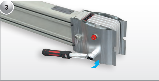
Blok ek somunları gevşetilir.
