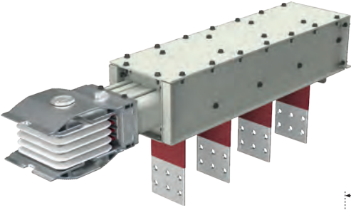
Yatay Pano/Trafo Modülü Pano/Trafo Çıkışı
