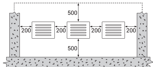
ŞEKİL 10 - GALERİ YATAY POZİSYON
