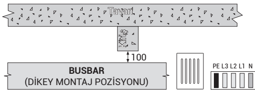
ŞEKİL 4 - KİRİŞ GEÇİŞİ DİKEY POZİSYON
