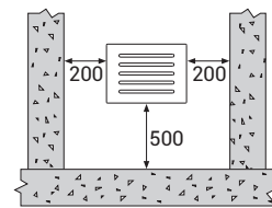
ŞEKİL 9 - GALERİ YATAY POZİSYON
