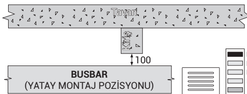
ŞEKİL 5 - KİRİŞ GEÇİŞİ YATAY POZİSYON
