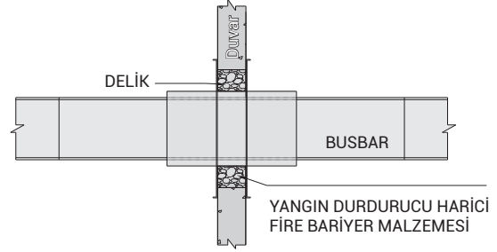
ŞEKİL 7 - STANDART DUVAR GEÇİŞİ
