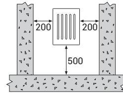
ŞEKİL 8 - GALERİ DİKEY POZİSYON
