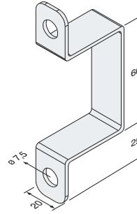
KA-TD Duvar Tespit Elemanı
