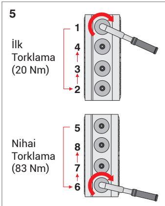
5- Busbar iki veya daha fazla yolluysa Şekil 5'deki gibi en kenardaki somunlar sıkılacak biçimde ilk önce 20 Nm ile daha sonra aynı sırayı takip ederek 83 Nm ile tork anahtarıyla sıkılır.
