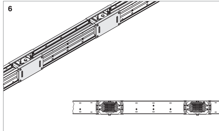
6- Ek yan kapakları da takılır. Kapak vidaları da takılarak montaj işlemi bitirilir. (15Nm)
