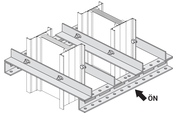
Dikey Şaft Uygulaması Kat Askı Örneği (Proje Özel)
